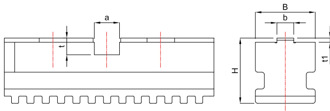
Grundbacken - Maßblatt
