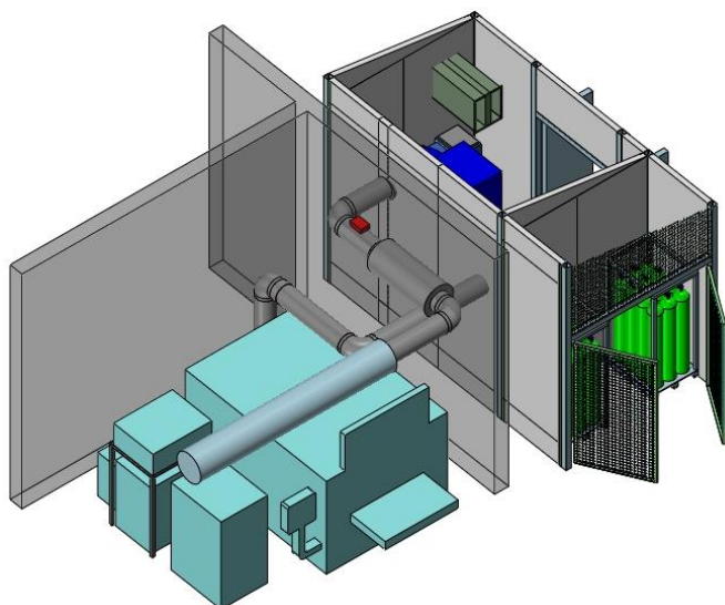
Abbildung: Aufstellungskonzept als Planungsgrundlage für die behördliche Einreichung und zur Raumplanung des Kunden in einem Ausbildungsbetrieb für einen Faserlaser SF1313 mit 1,5 KW. Inklusive aller Komponenten, Gaslager für Sauerstoff und Stickstoff, inklusive Schall- und Wärmeschutz-Einhausung für die Absaugung und den Kompressor.
